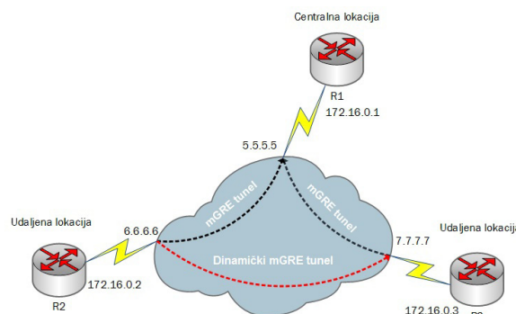
Slika 4. Prikaz DMVPN tunela
